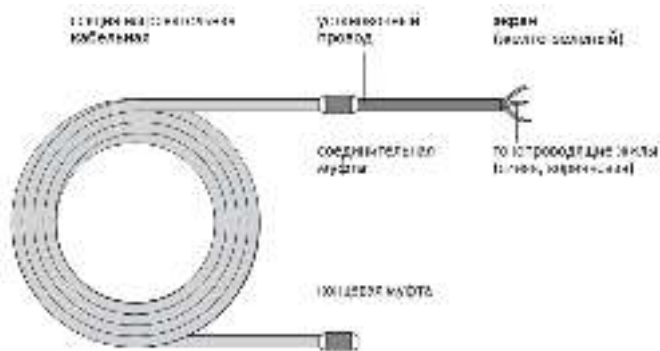
Рис. 1 - Конструкция секции нагревательной кабельной Freezstop Inside Dachha
